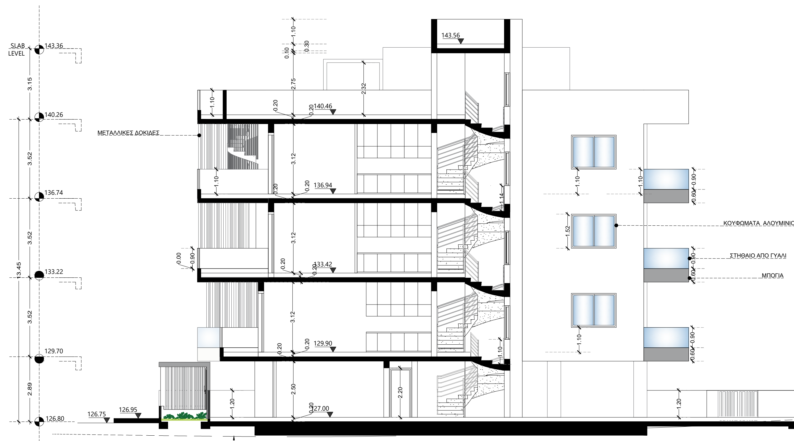
ΤΟΜΗ Γ-Γ
