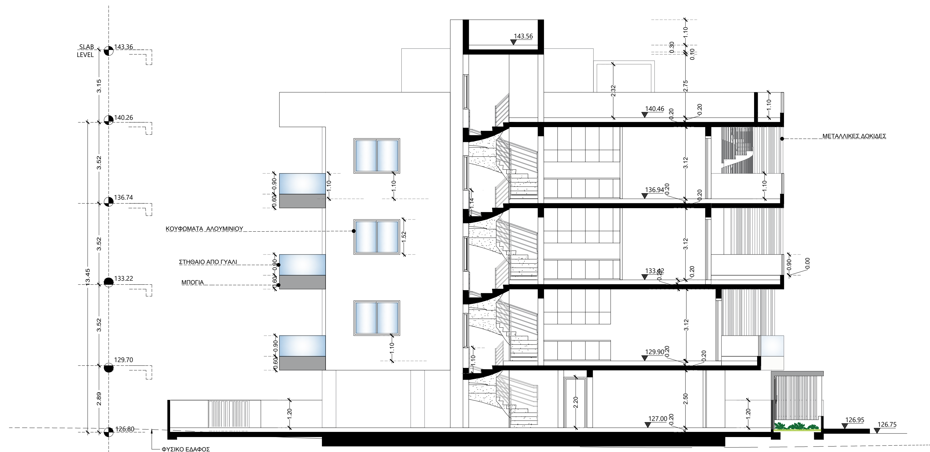
ΤΟΜΗ Α-Α
