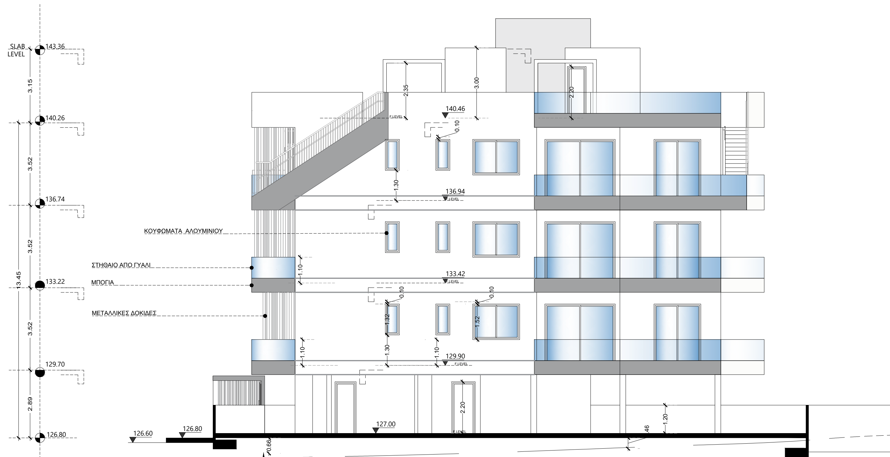
ΠΛΑΓΙΑ ΟΨΗ Ε2
