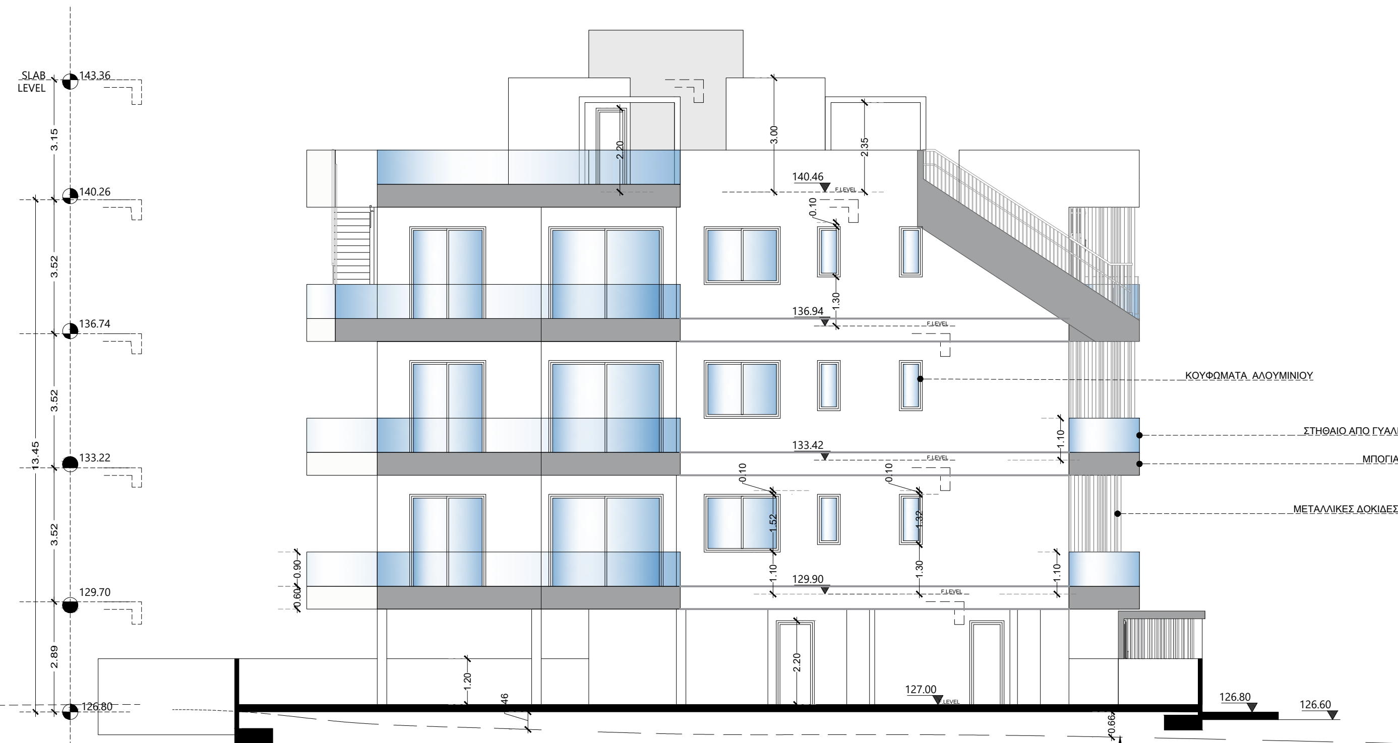
ΠΛΑΓΙΑ ΟΨΗ Ε4
